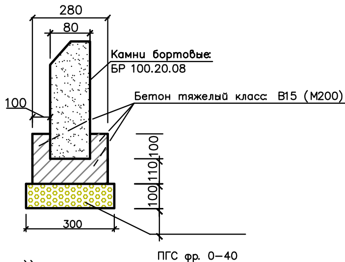
Узел бортового камня БР 100.20.8
