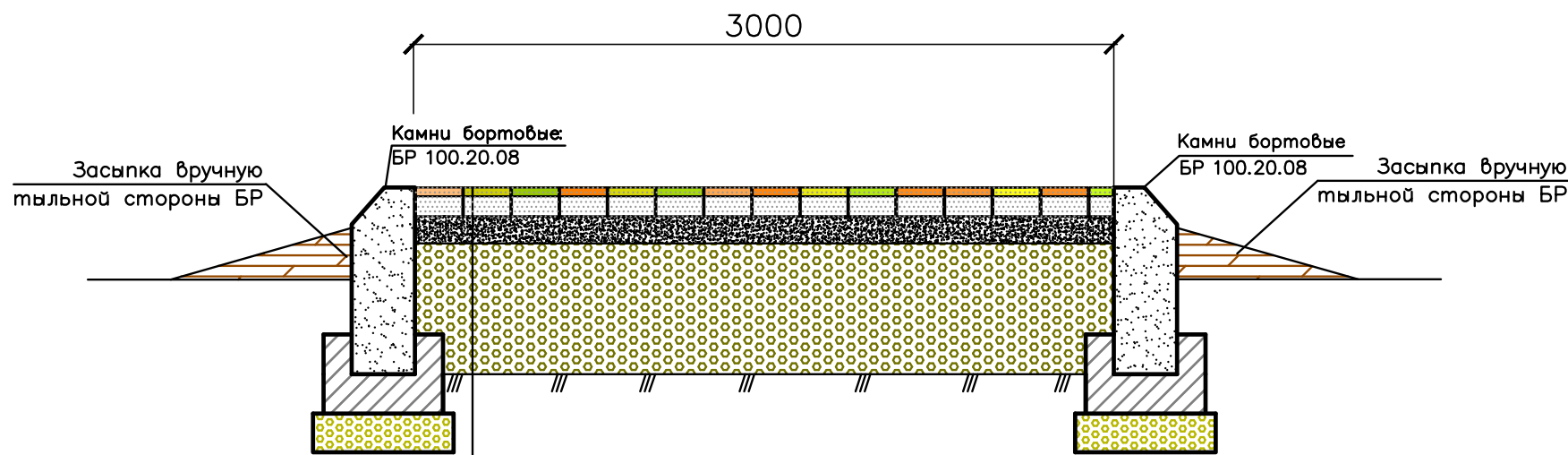
Конструкция тротуара Разрез 1-1
