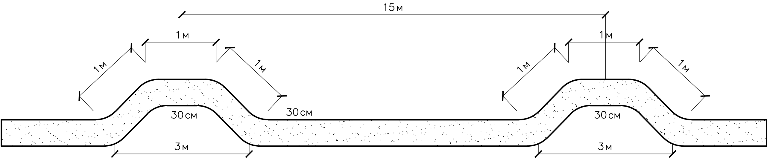
Схема велосипедной дорожки
